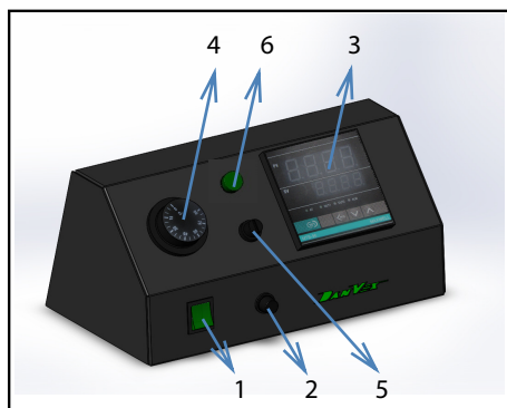
Рис. Пульт управления котлом.
