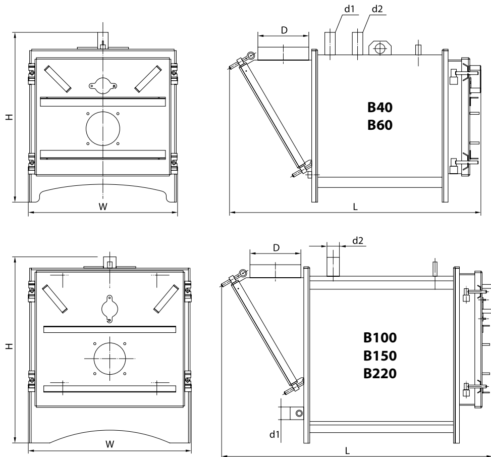
Рис. 3 Габариты котлов
