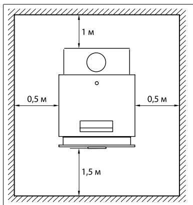
Рис. 4 Минимальные расстояния от стен
